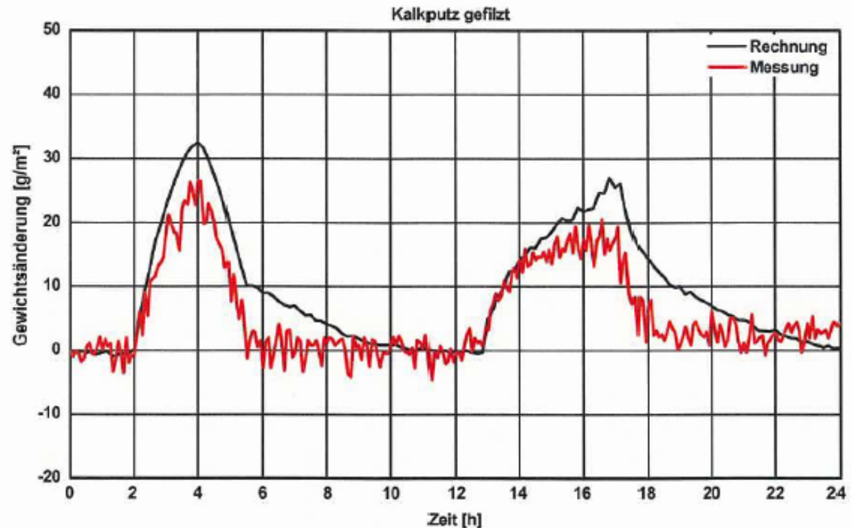
Bild 14: Vergleich der gemessenen und berechneten Verläufe der Gewichtsänderung beim Laborversuch mit Kalkputz mit Kalkputz mit gefilterter Oberfläche über einen Zeitraum von 24 Stunden.
