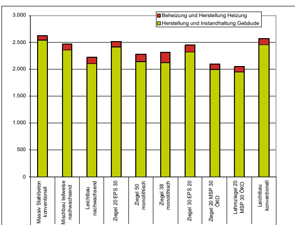
Abb. 3: Versauerungspotential des Gebäudes mit Erdgasheizung in [kg SO 2 äquiv.]
