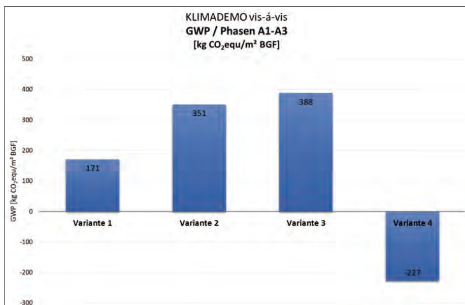
Abb. 2: Treibhauspotential (GWP) der vier Varianten für das Bauprojekt vis-à-vis im Village im Dritten für das gesamte Gebäude. Variante 1: Plan vis-à-vis, Variante 2: Beton Skelett, Variante 3: Beton massiv, Variante 4: best case. Die Berechnungen erfolgten mit dem Tool eco2soft, berücksichtigt wurden die Phasen A1 bis A3 (Herstellungsphase) gemäß EN 15978. Bei der Berechnung berücksichtigt wurden sämtliche Bauteile (exkl. Haustechnik).
