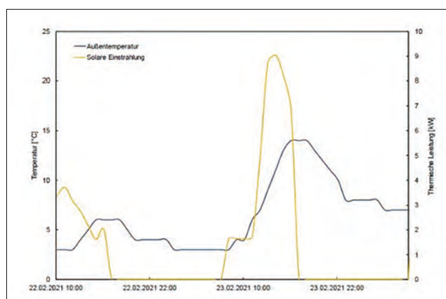
Abb. 2: Basiswetterdaten Sonnenstrahlung / Außentemperatur: Die Wetterdaten zeigen, dass in 24 Stunden ein schöner und sonniger Tag wird.
