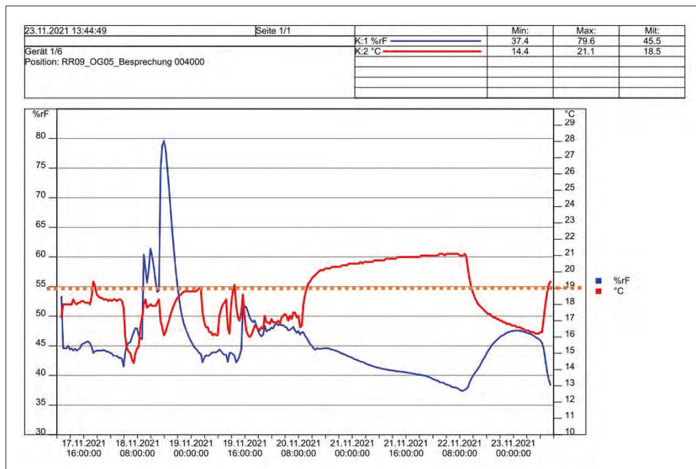
Abb. 10: Ergebnisse der Raumluftfeuchte- und Raumlufttemperaturmessung im Rahmen des baubegleitenden Feuchte-Monitorings. Durch Beheizung wird kritische Feuchtespitze wieder abgesenkt.
