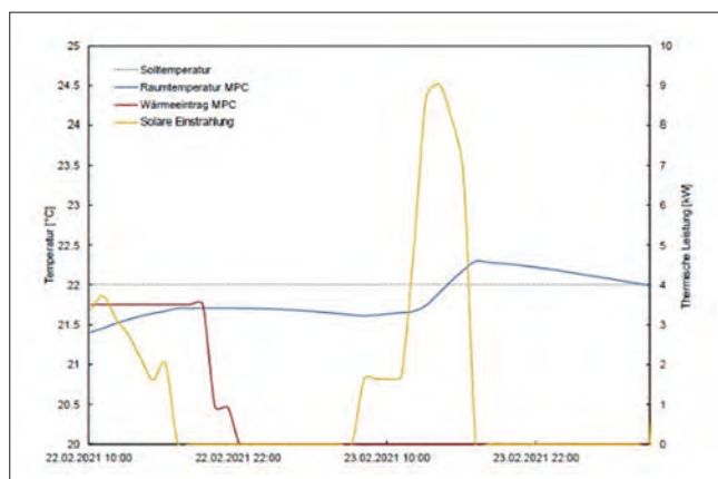
Abb. 3: Die prognosebasierte Steuerung erkennt, dass mit den solaren Erträgen die Wunschttemperatur erreicht werden kann und reduziert bereits 14 Stunden vorher am Abend des Vortages (22.02.2021 um 22:00 Uhr) den Wärmeeintrag.
