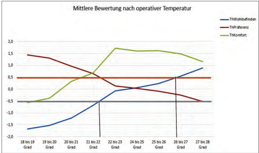
Abb. 3: Mittlere Bewertung für die Variablen ThWohlbefinden (Fanger-Skala), ThPräferenz und ThKomfort (Behaglichkeit)
